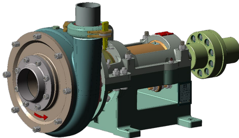
Углесосы У900-90М, У900-120, У900-180 (присоединительные размеры)
