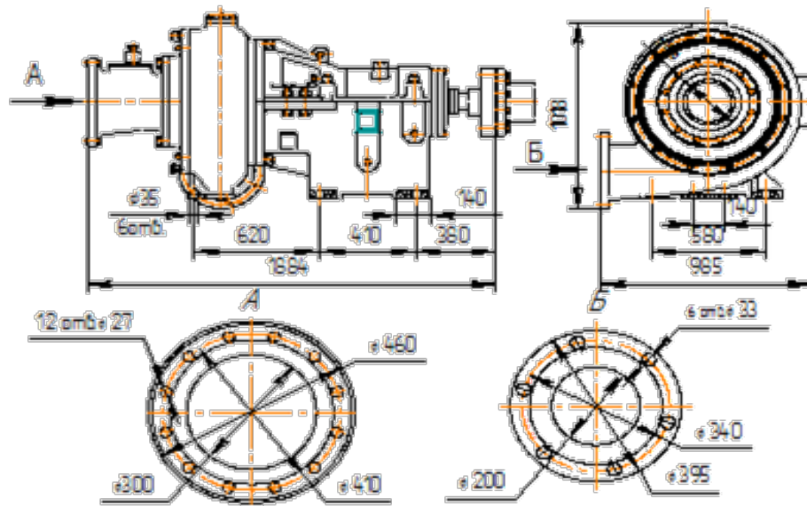
Углесосы У450-60, У450-80, У450-120, У450-160 (присоединительные размеры)
